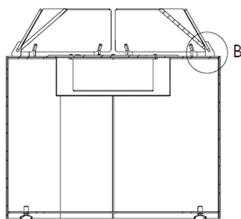
SEZIONE A-A
